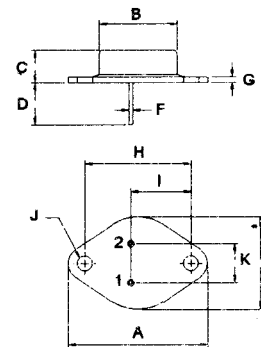
TO-3
